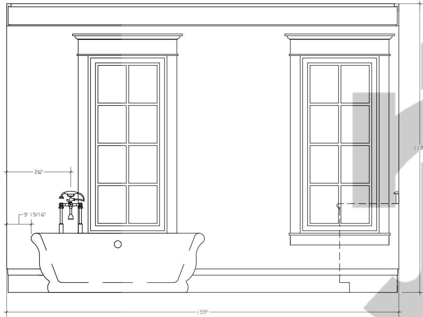
3 MASTER BATH ELEVATION SCALE: 1/2" = 1'-0"
