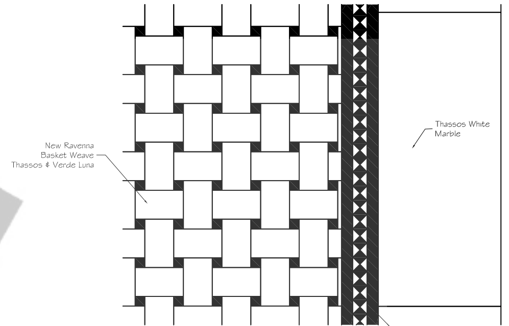
4 TILE DETAIL SCALE: 3" = 1'-0"
